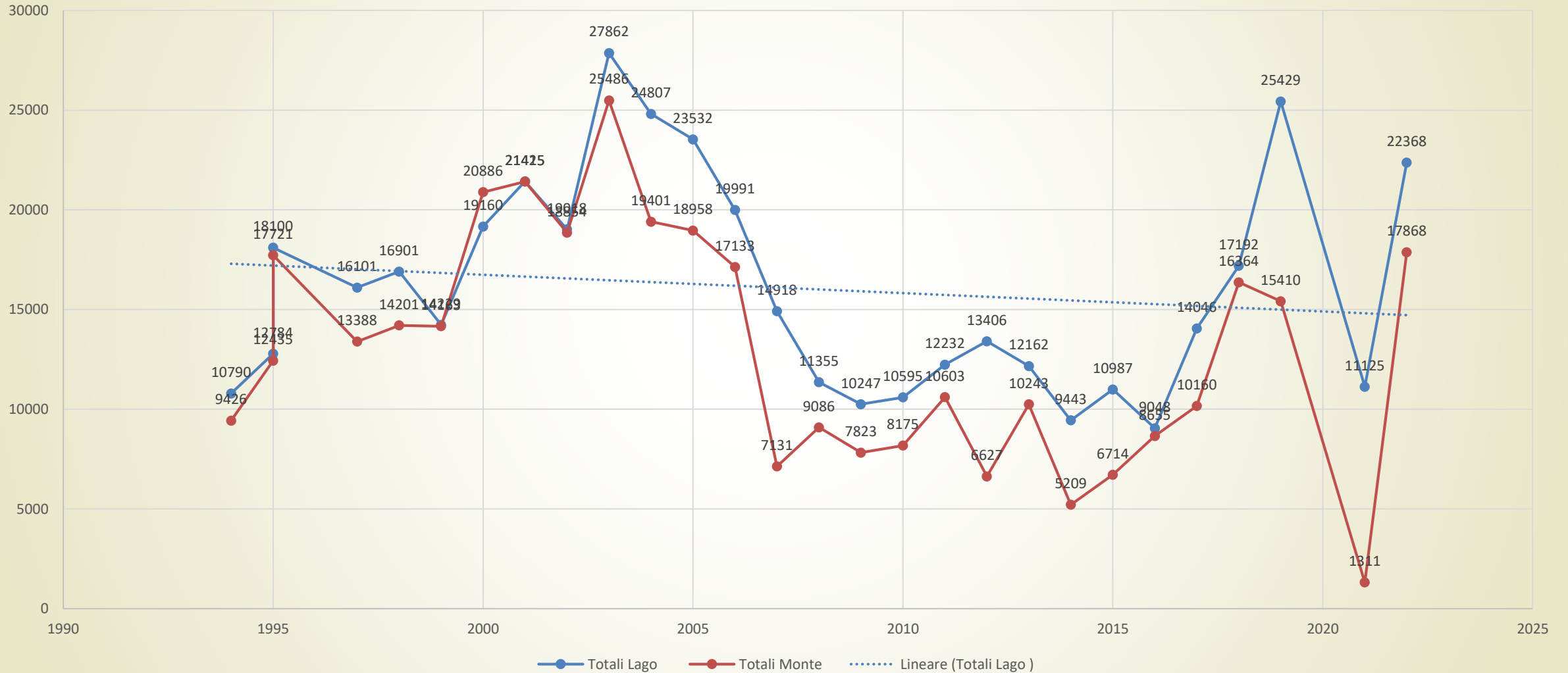
Andamento consistenza popolazione di rospo comune (Bufo bufo)
