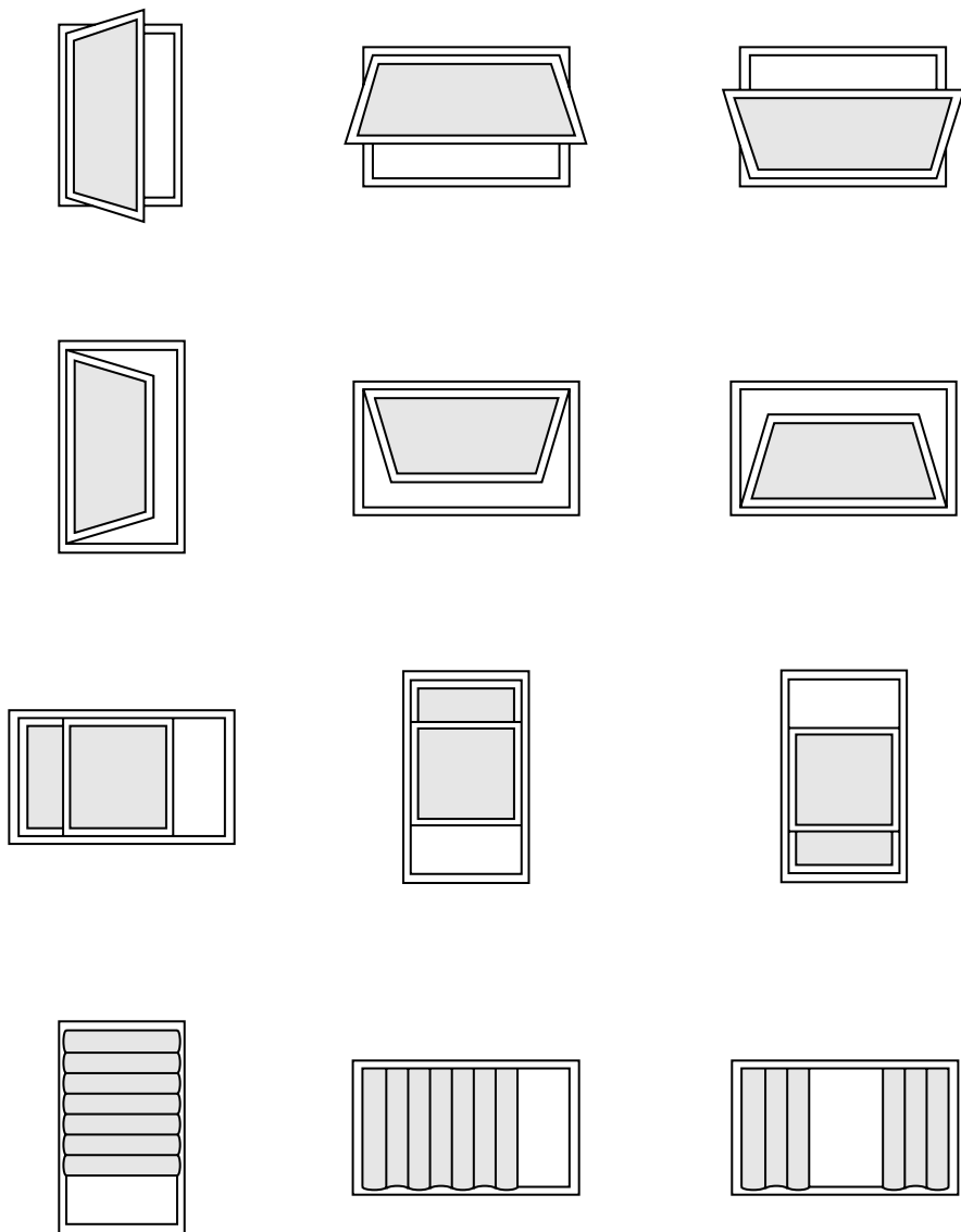
Esempi di diversi tipi di chiusura per le aperture: ante battenti verso l'interno o verso l'esterno, ante scorrevoli e tende oscuranti. Gli schemi delle ante possono essere applicati sia ai sistemi oscuranti (per esempio, pannelli di legno) sia alle chiusure vetrate. Per queste ultime è bene sia prevista l'aggiunta di tende oscuranti.
